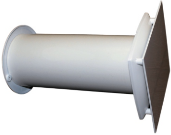
Рекуператор «Салюс ТкV-01H/200 Крым»
